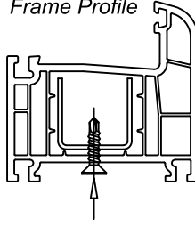
Ø 3,9 x 16 YHB matkap uçlu vida / screw
