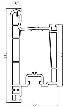
606 Dışa Açılır Kapı Profili Outside Opening Door Profile 1,730 kg/m
