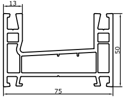
751 Sürme Kasa Sliding Frame 1,280 kg/m
