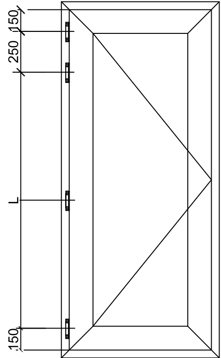
Kapı Kanadı / Door Sash
