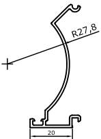
6507 Eksenel Dönüş Adaptörü Corner Pipe Adaptor Profile 0,350 kg/m (Al) / 0,400 kg/m (PVC)
