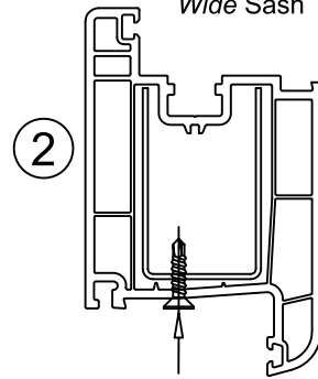
Ø 3,9 x 16 YHB matkap uçlu vida / screw
