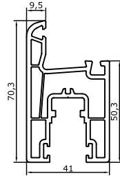
793 Sürme Kanat Sliding Sash Profile 0,960 kg/m
