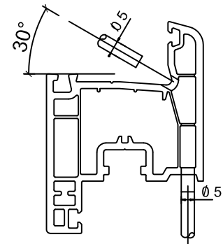
Su Tahliye Kapağı Water Exit Cap
