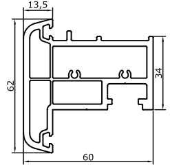
604 Hareketli Orta Kayıt Overhang Profili 1,105 kg/m
