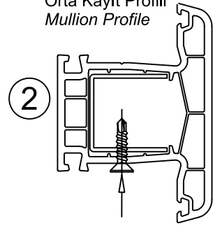
\text{Ø } 3,9 \times 16 YHB matkap uçlu vida / screw
