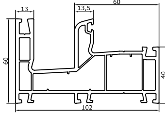
755 Sürme Fiks Kasa Fix Sliding Frame 1,625 kg/m
