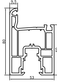
752 Sürme Kanat Sliding Sash 1,400 kg/m
