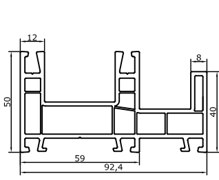
791 Sürme Sineklikli Kasa 3 Track Sliding Frame Profile 1,350 kg/m
