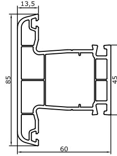
632 Orta Kayıt Mullion Profili 1,100 kg/m
