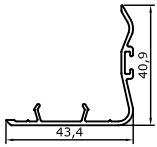
796 Sürme Kanat Kapama (interlok) Interlock Profile 0,185 kg/m
