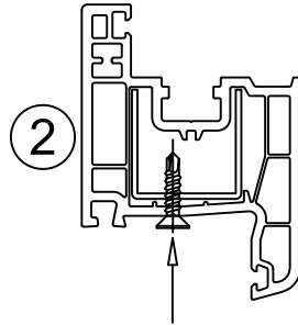
\text{Ø } 3,9 \times 16 YHB matkap uçlu vida / screw
