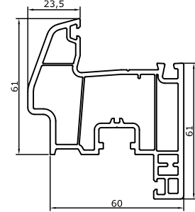
703 Damlalıklı Kanat Profili Wide Sash Profile 1,230 kg/m
