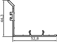
6505 Sürme Kenet Profili Interlock Profile 0,455 kg/m
