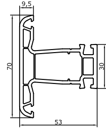
753 Sürme Orta Kayıt Sliding Mullion 0,905 kg/m
