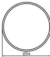
613 Eksenel Dönüş Borusu Corner Pipe Profile 0,680 kg/m (Al) / 0,800 kg/m (PVC)
