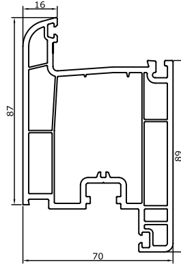
7005 Kapı Kanat Profili Door Sash Profile 1,700 kg/m
