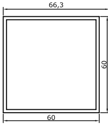
916/B Köşe Dönüş Kutu Profili Corner Box Profile 1,270 kg/m (Al) / 0,800 kg/m (PVC)
