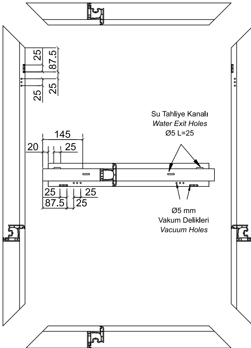
Vakum Delikleri Vacuum Holes
