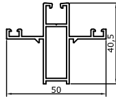
6511 Birleşim Adaptörü Connection Profile 0,620 kg/m
