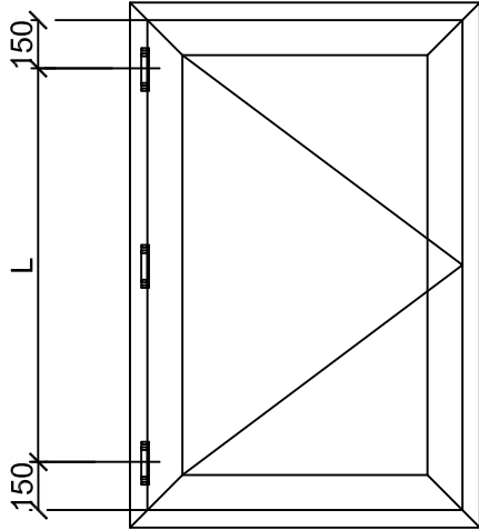
Pencere Kanadı / Window Sash
