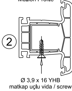
Orta Kayıt Profili Mullion Profile
