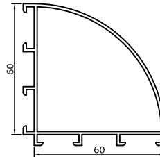
4186 90° Dönüş Profili 90° Corner Profile 1,020 kg/m
