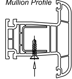
Ø 3,9 x 16 YHB matkap uçlu vida / screw
