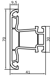
792 Sürme Orta Kayıt Sliding Mullion 0,735 kg/m
