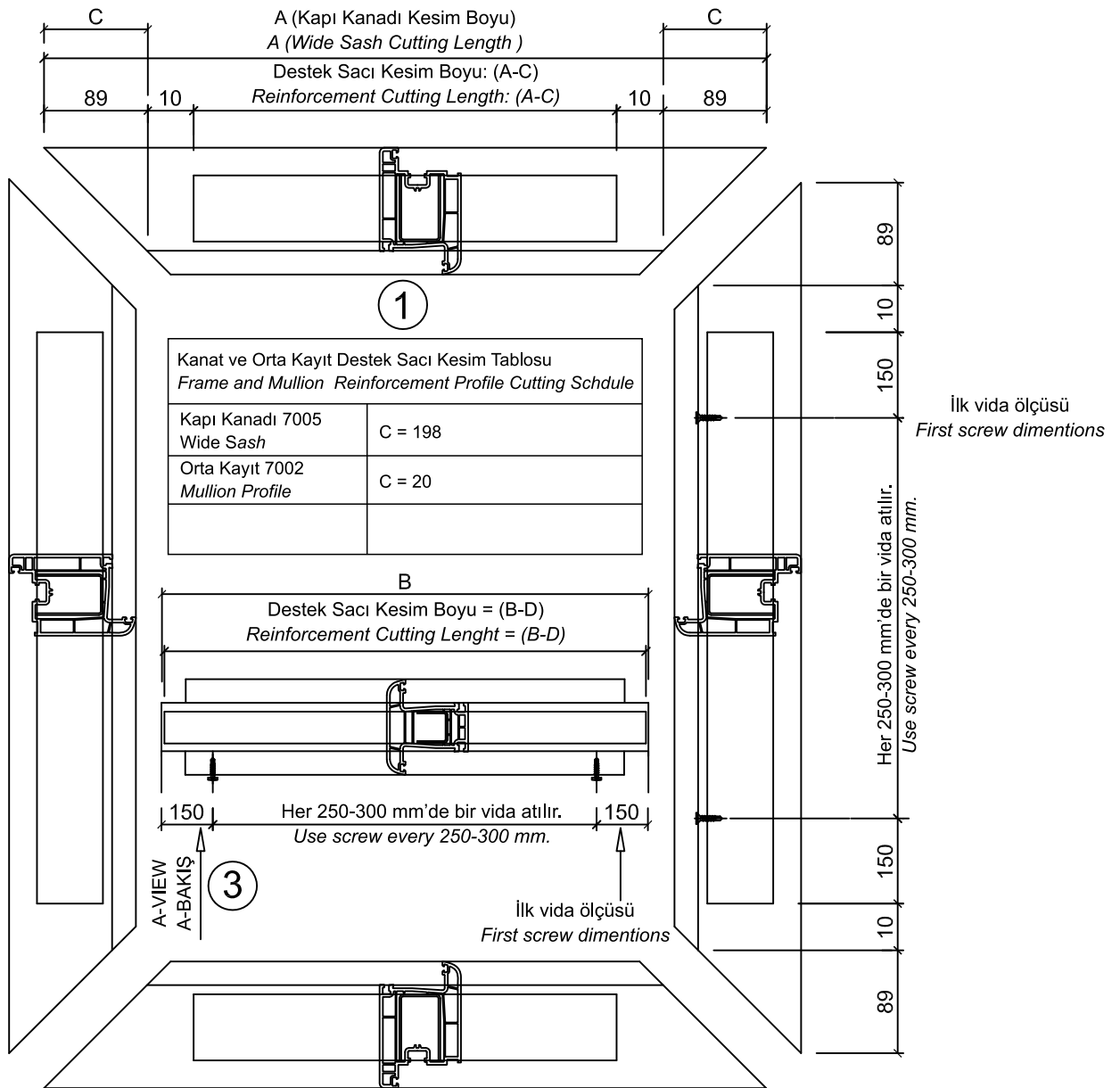
Ø 3,9 x 16 YHB matkap uçlu vida / screw
