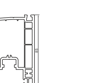
407 Dış Kapa Kanat Profil Tight Door Sash Profile 1.485 kg/m
