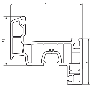
7404 Dar Kanat Profil Tight Sash Profile 1.334 kg/m 7411 Hareketli Orta Kayıt Profil Overhang Profile 1.256 kg/m
