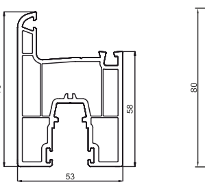
758 Pervazlı Sinekli Kasa Sliding Frame 1.860 kg/m
