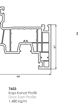
7603 Kapa Kanat Profil Door Sash Profile 1.480 kg/m 7605 Dış Açılır Kapa Profil Outside Opening Door Profile 1.760 kg/m
