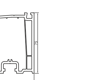
606 Dış Açılır Kapa Profil Outside Opening Door Profile 1.720 kg/m
