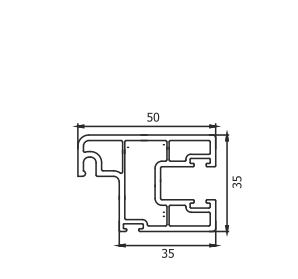
752 Sürme Kanat Sliding Sweater Sash 0.638 kg/m 753 Sürme Orta Kayıt Sliding Mullion 0.890 kg/m
