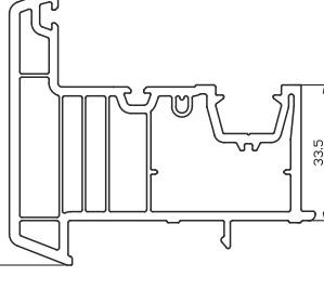
7410 Dar Hareketli Orta Kayıt Profil Tight Overhang Profile 1.056 kg/m 7412 Sürme Ekonomik Kanat Sliding Sweater Sash 1.1151 kg/m
