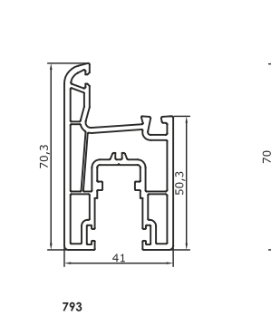
792 Sürme Orta Kayıt Sliding Mullion 0.715 kg/m 795 Sürme Sinekli Kanat Sliding Sweater Sash Profile 0.310 kg/m
