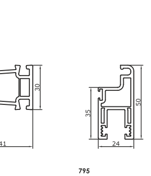
794 Sürme Sinekli Orta Kayıt Sliding Sweater Mullion Profile 0.369 kg/m 794 (4518) Sürme Kanatı Kapama (İnterlok) Interlock Profile 0.380 kg/m
