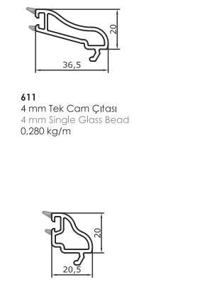
605 Kapa Kanat Profil Door Sash Profile 1.680 kg/m 604 Hareketli Orta Kayıt Overhang Profile 1.053 kg/m
