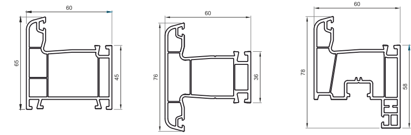
651 Ekonomik Düz Kasa Profil Economic Flat Frame Profile 0.835 kg/m 652 Ekonomik Orta Kayıt Profil Economic Mullion Profile 0.876 kg/m 653 Ekonomik Kanat Profil Economic Sash Profile 1.000 kg/m 703 Dönme Kanat Profil Wide Sash Profile 1.170 kg/m
