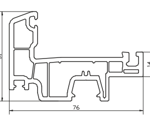
7602 Orta Kayıt Profil Mullion Frame Profile 1.410 kg/m 7604 Dar Kanat Profil Tight Sash Profile 1.334 kg/m
