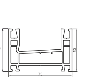
751 Sürme Kasa Sliding Frame 1.250 kg/m 754 Pervazlı Sürme Kasa Wide Sliding Frame 1.170 kg/m
