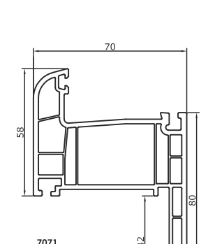
7021 Ekstrem Dönme Bonusu Corner Pipe 0.780 kg/m 7022 Ekstrem Dönme Adaptörü Corner Pipe Adapter 0.450 kg/m 7005 Kapa Kanat Profil Door Sash Profile 1.690 kg/m 7006 Dış Açılır Kapa Kanat Profil Outside Opening Door Sash 1.730 kg/m
