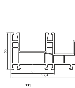
791 Sürme Sinekli Kasa 3 Track Sliding Frame Profile 1.310 kg/m 793 Sürme Kanat Sliding Sash Profile 0.935 kg/m
