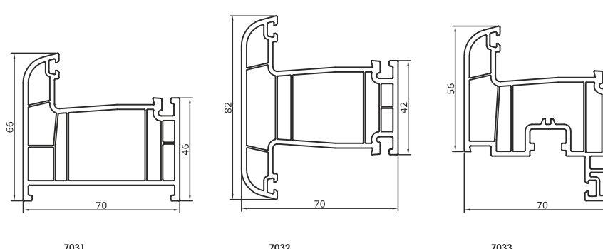
701 Kasa Profil Frame Profile 1.040 kg/m 702 Orta Kayıt Profil Mullion Profile 1.145 kg/m 703 Kanat Profil Sash Profile 1.225 kg/m 707 Pervazlı Kanat Profil Wide Frame Profile 1.222 kg/m
